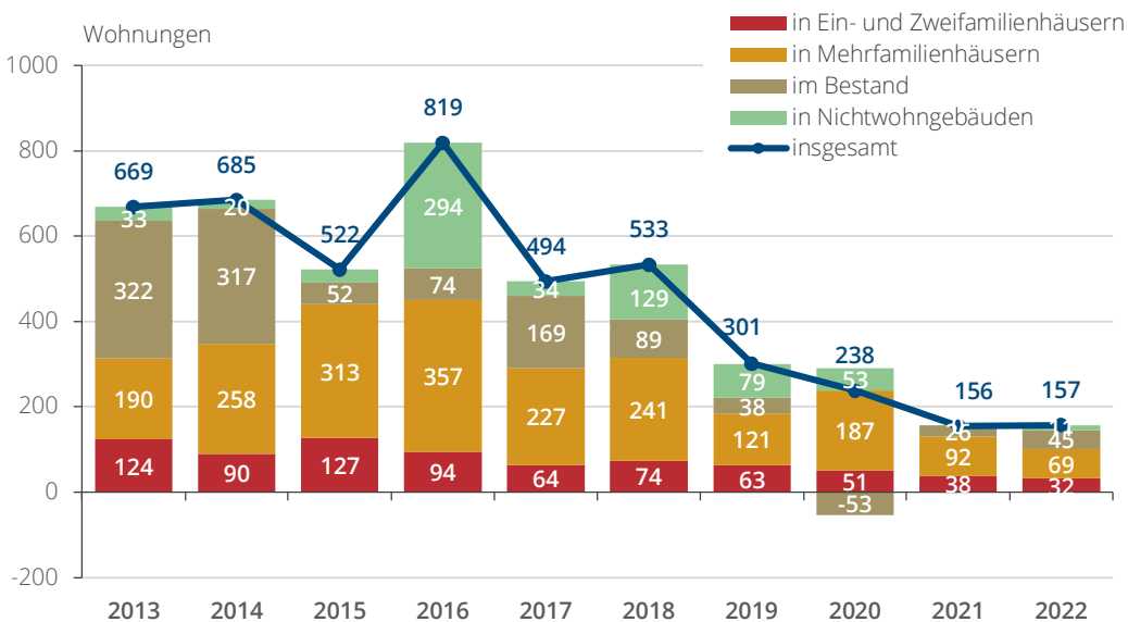
ABB. 3 BAUFERTIGSTELLUNGEN IN JENA 2013 BIS 2022
